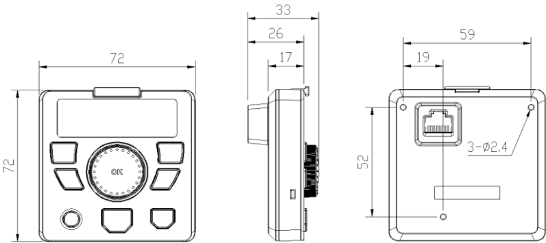
图 C-1 单显外引键盘安装尺寸（单位：mm）
