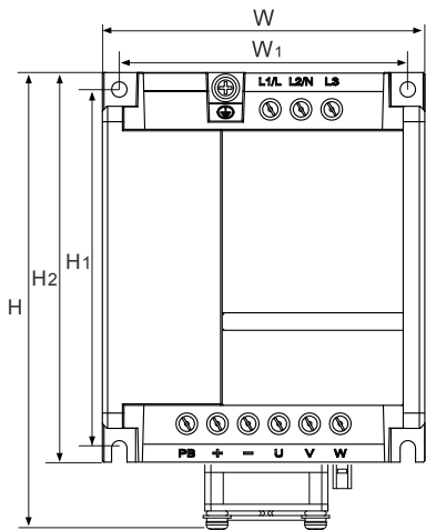
图 2-4 壁挂式安装示意图
