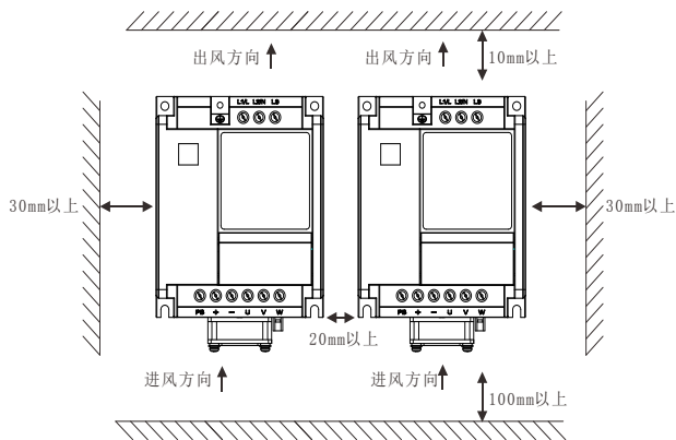
图 2-3 两台变频器左右安装
