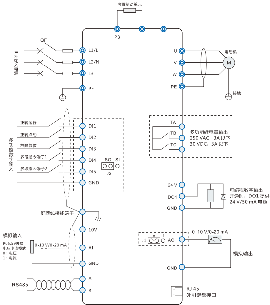
图 2-6 M100 系列变频器系统配线图
