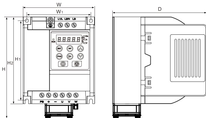
图 C-6 框架 A/B 安装尺寸
