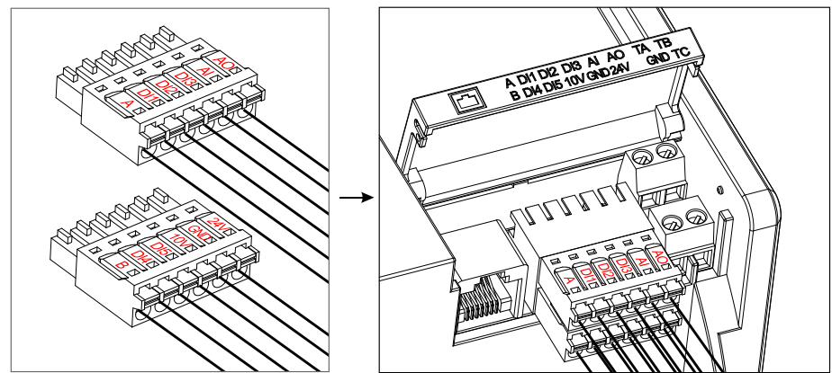
图 2-5 端子安装示意图
